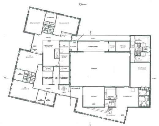
VOORONTWERP - plattegrond
